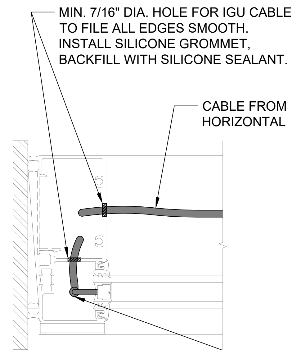
DETAIL 4 LEFT JAMB
